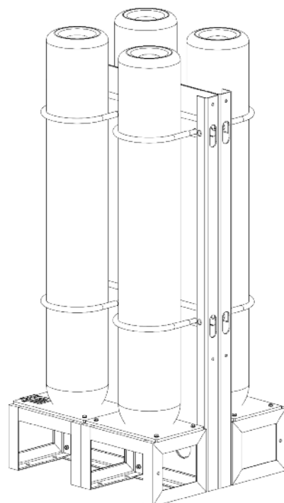
#ASCR320-350 HOCHDRUCKSPEICHER STORAGE CYLINDER RACK
