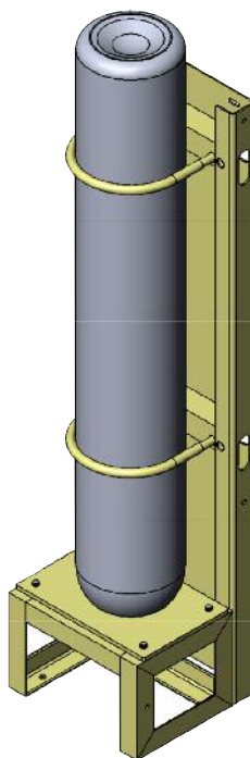
#ASCR50-350 HOCHDRUCKSPEICHER STORAGE CYLINDER RACK
